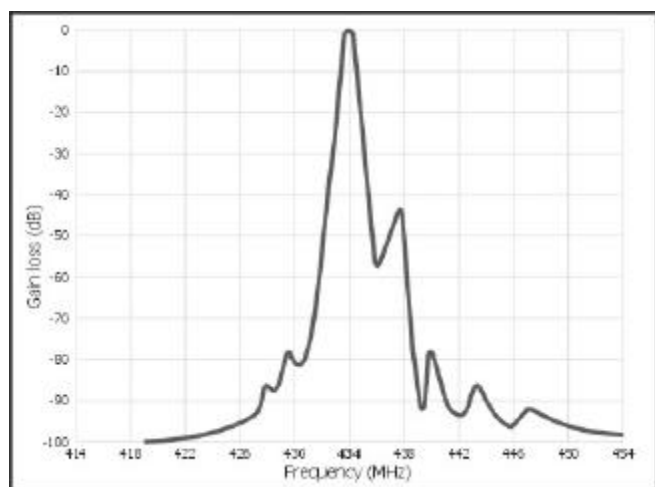
Fig.4 Grafico Frequenza-Selettività
